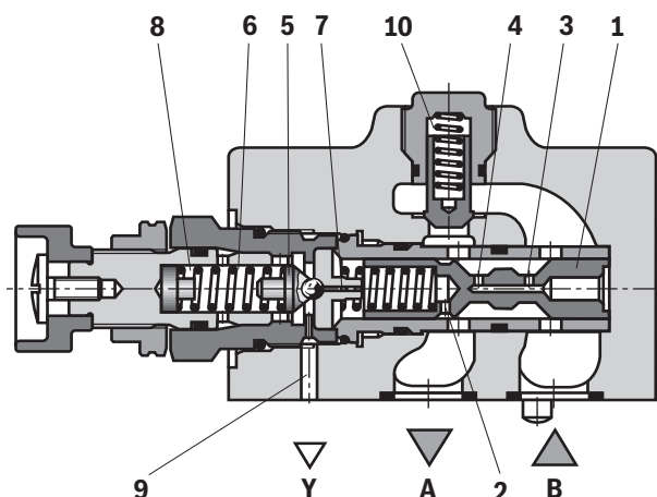
Type DR 10 -4-4X/...
