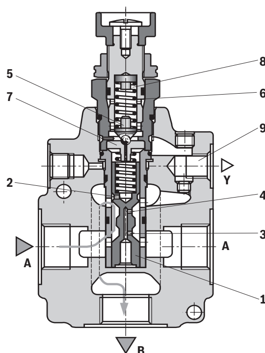
Type DR 20 G-4-4X/...
